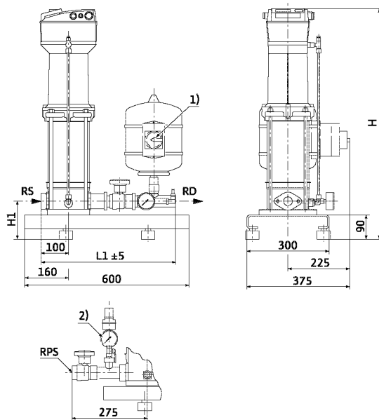
Габаритный чертеж
