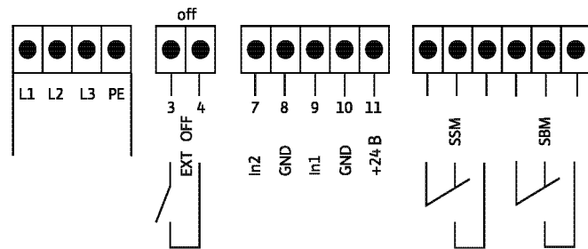
Схема подключения
